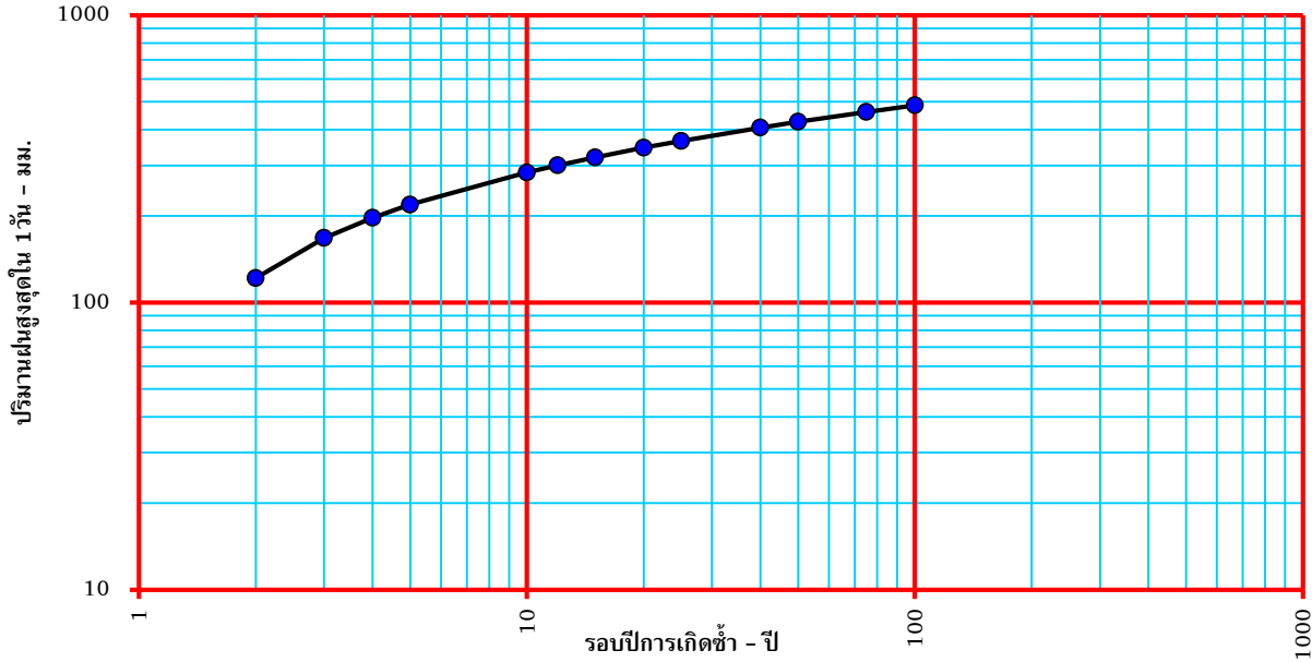
แสดงรอบปีการเกิดซ้ำปริมาณฝนสูงสุดใน 1 วัน สถานี 450371 (ต่งไม้้งาม) ต.ชัยเกษม อ.บางสะพาน จ.ประจวบคีรีขันธ์
