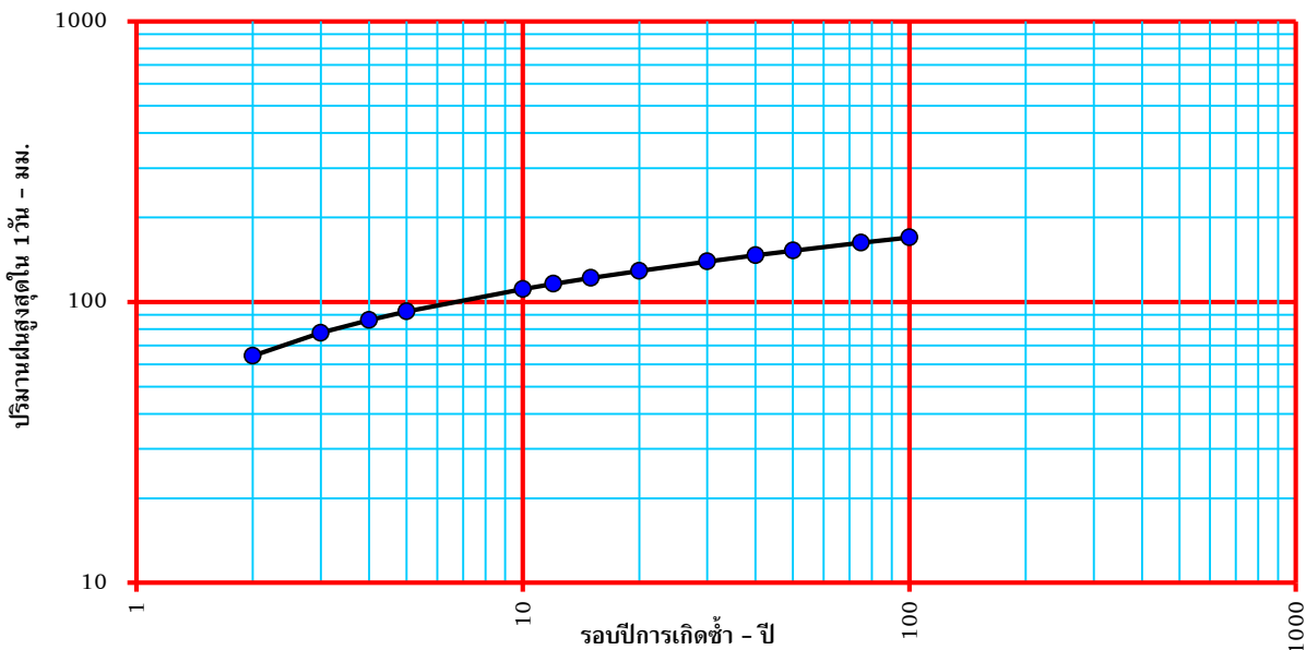
แสดงรอบปีการเกิดซ้ำปริมาณฝนสูงสุดใน 1 วัน สถานี 370411 (FP.02) อต.ห้วยกระสังข์ อ.แก่งกระจาน จ.เพชรบุรี
